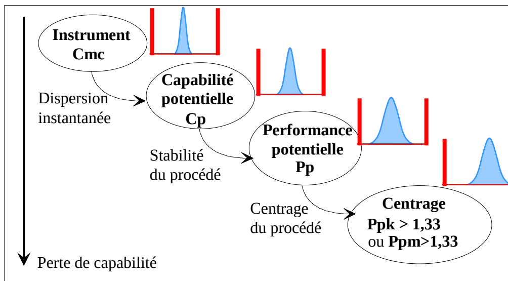
figure 4 – Chute de capacité du Cmc vers le Ppk/Ppm
